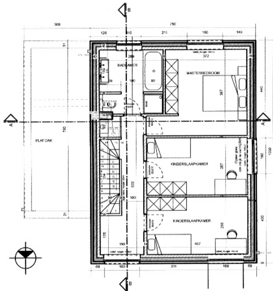
WONING 1 - 1ste VERDIEPING
